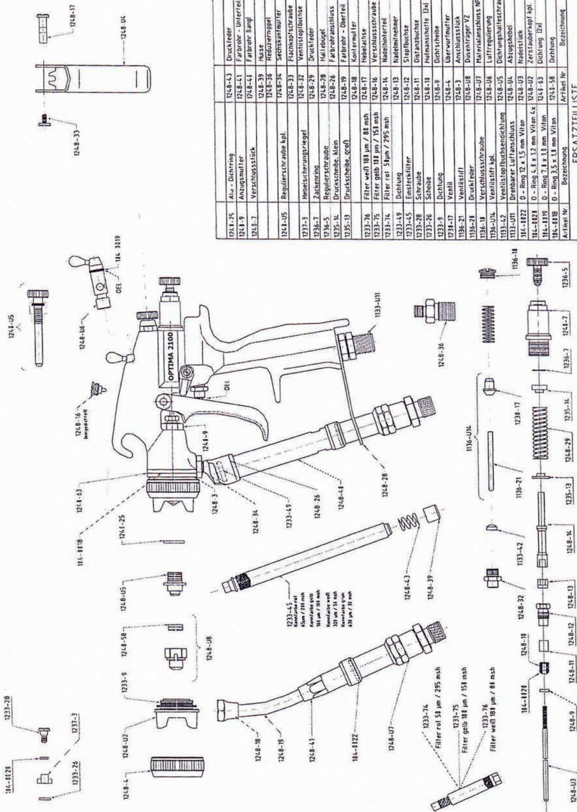
Abbildung 4: Explosionszeichnung der Optima 2100
